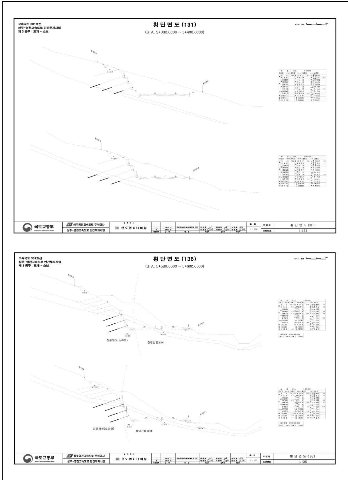
【그림 16.1.5】 표준횡단면도
